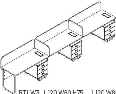
RTLW3 L120 W60 H75 L120 W80 H75 L140 W60 H75 L140 W80 H75 L160 W60 H75 L160 W80 H75
