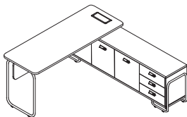
Side L189 RTDS4 L180 W60 H75 L180 W80 H75 L200 W60 H75 L200 W80 H75
