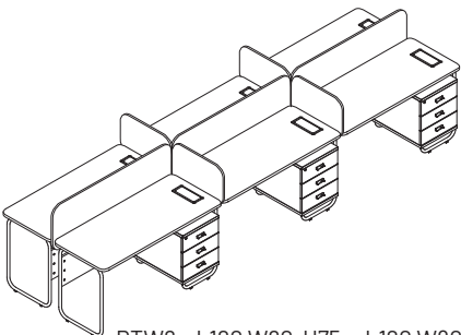
RTW6 L120 W60 H75 L120 W80 H75 L140 W60 H75 L140 W80 H75 L160 W60 H75 L160 W80 H75
