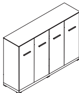
CLCW L184 W43 H125
