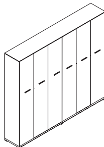
CLCW L274 W43 H164
