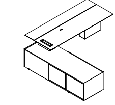
VISU R/L VIDV 60 R/L L230 W76 H64 L200 W100 H75 L260 W100 H75 L220 W100 H75 L280 W100 H75 L240 W100 H75
